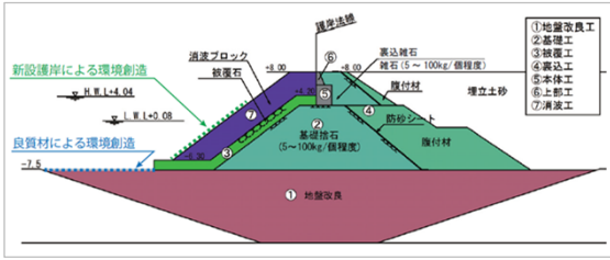
主な護岸の標準断面図（南・東護岸）
