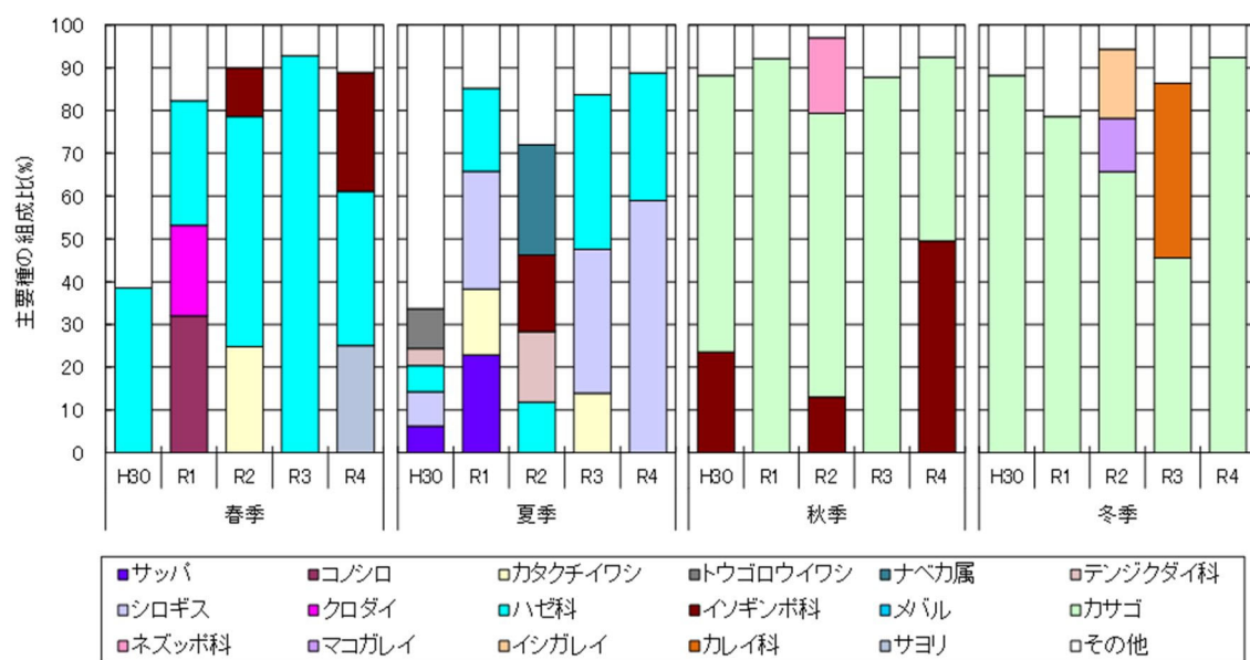
図 2.2.30 主な出現種の経年変化（稚仔魚）
