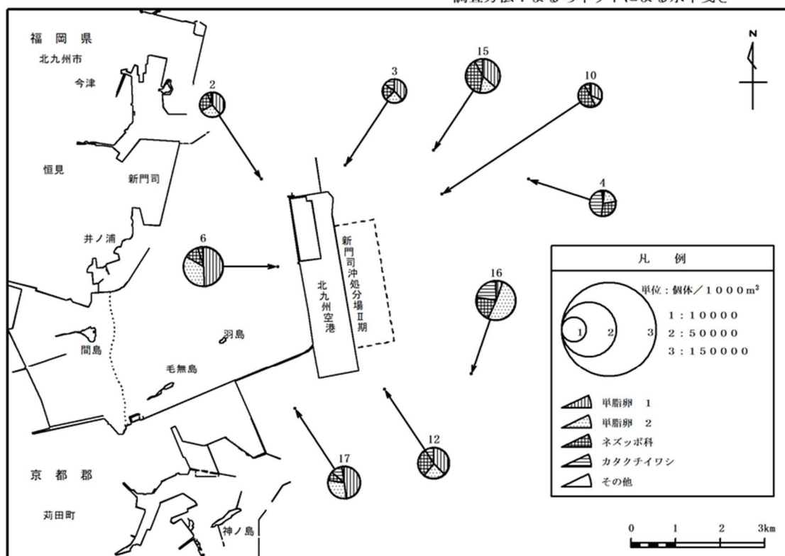
図 2.2.24(1) 魚卵の水平分布（令和 4 年度春季）
