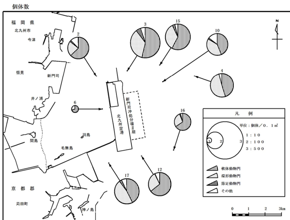
図 2.2.33(1) 底生生物の水平分布（令和 4 度春季：種類数・個体数）
