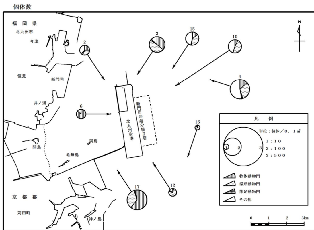
図 2.2.33 (3) 底生生物の水平分布（令和 4 年度秋季：種類数・個体数）
