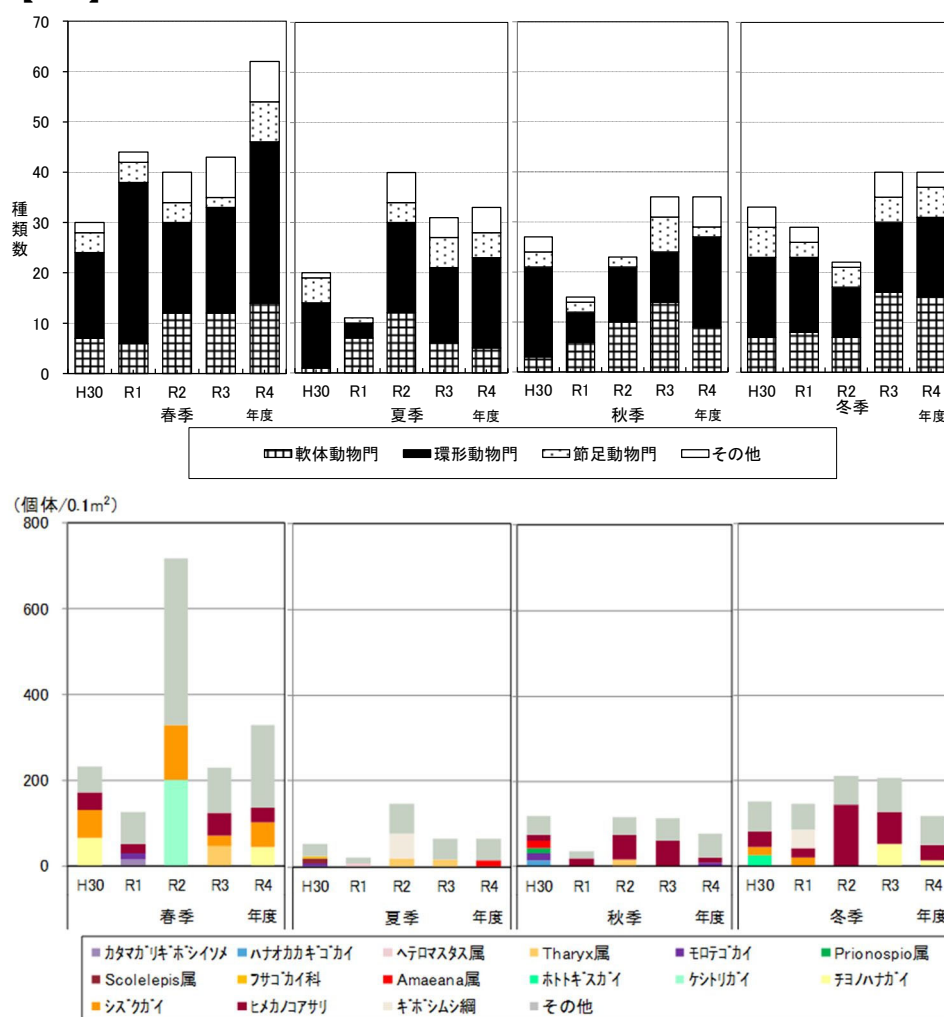
図 2.2.34(2) 底生生物の経年変化 (No. 3)
