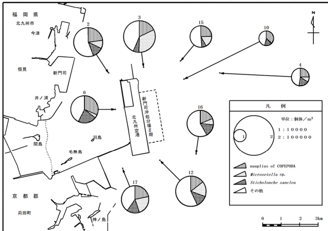
図 2.2.20(3) 動物プランクトンの水平分布（令和 4 年度秋季）
