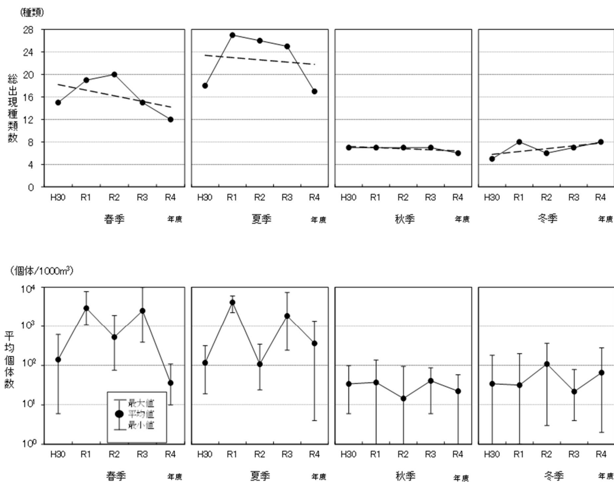
図 2.2.29 稚仔魚の経年変化
