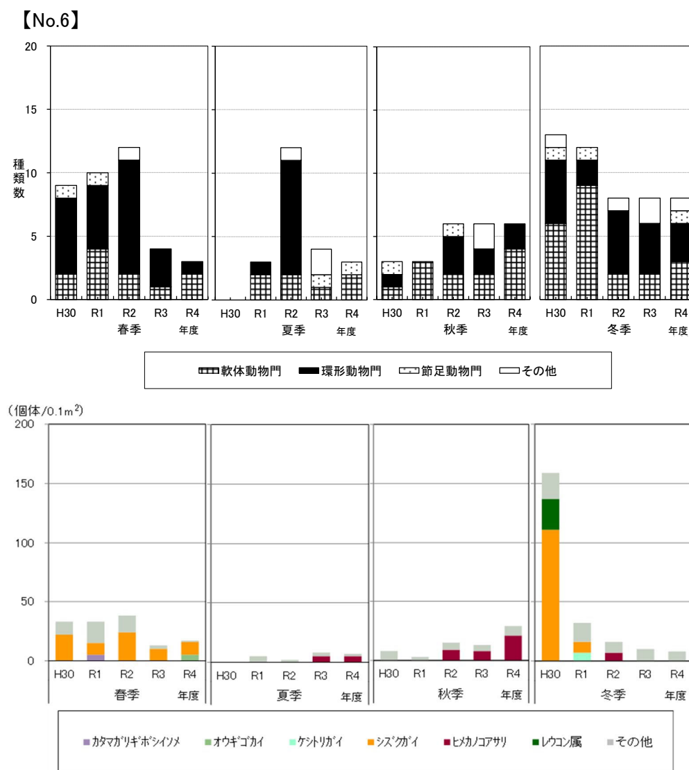
図 2. 2. 34(4) 底生生物の経年変化 (No. 6)
