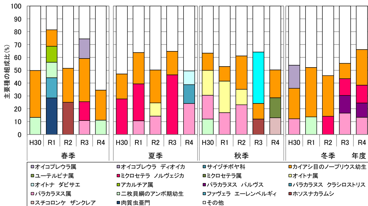
図 2.2.21 動物プランクトンの経年変化
