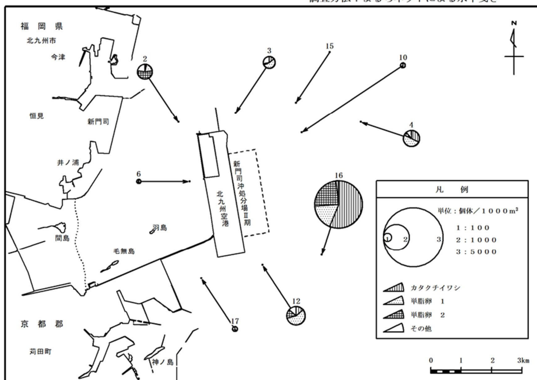
図 2.2.24(2) 魚卵の水平分布（令和 4 年度夏季）
