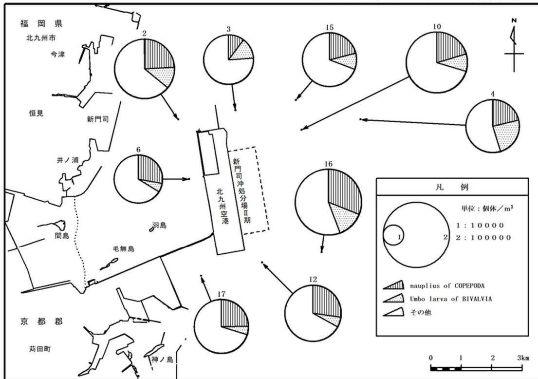
図 2.2.20(1) 動物プランクトンの水平分布（令和 4 年度春季）
