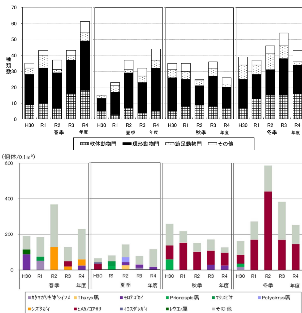
図 2. 2. 34 (9) 底生生物の経年変化 (No. 17)
