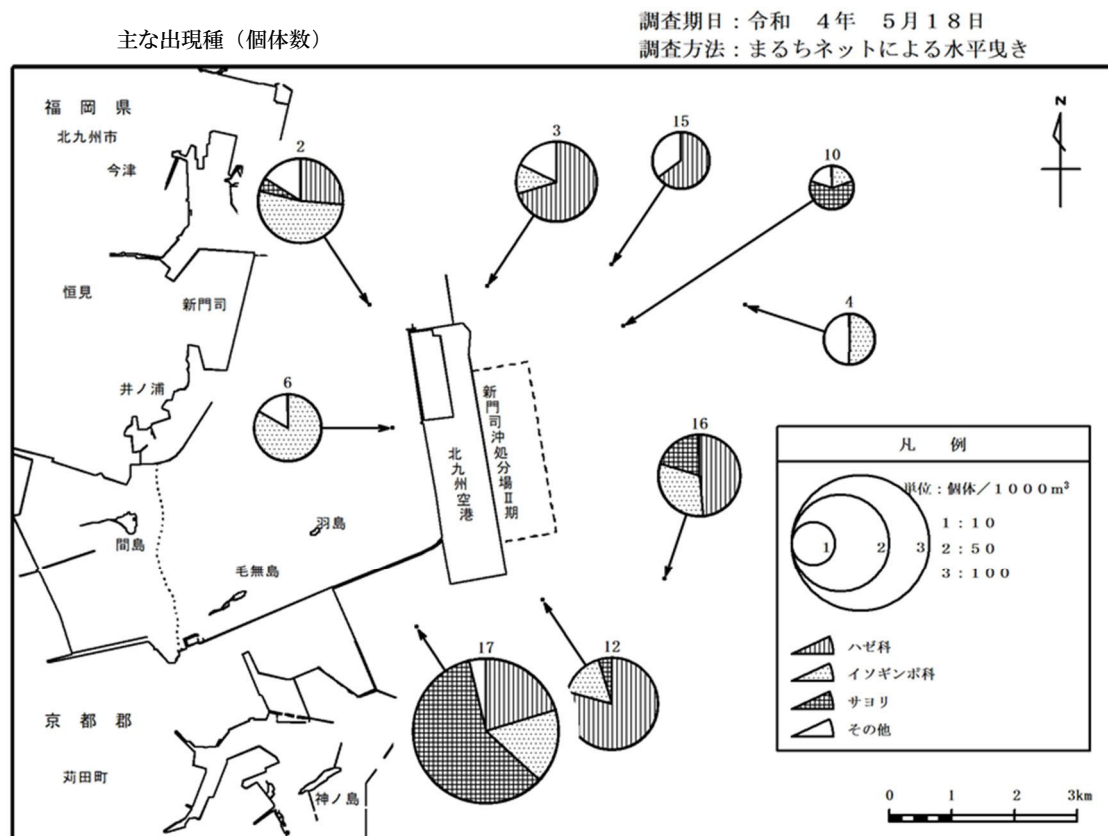
図 2.2.26(1) 稚仔魚の水平分布（令和 4 年度春季）
