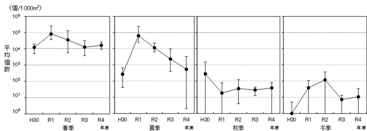
図 2.2.27 魚卵の経年変化
