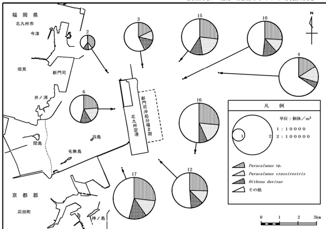
図 2.2.20(2) 動物プランクトンの水平分布（令和 4 年度夏季）
