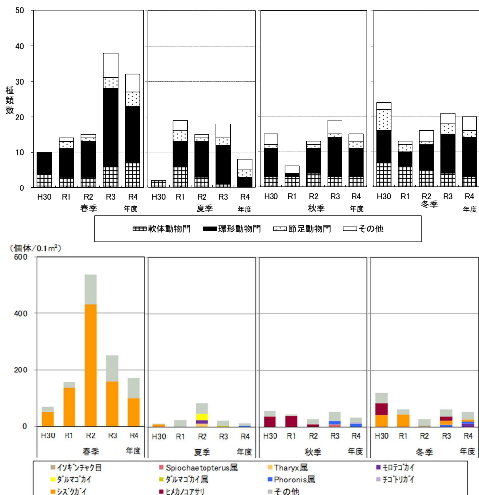
図 2.2.34(1) 底生生物の経年変化 (No. 2)
