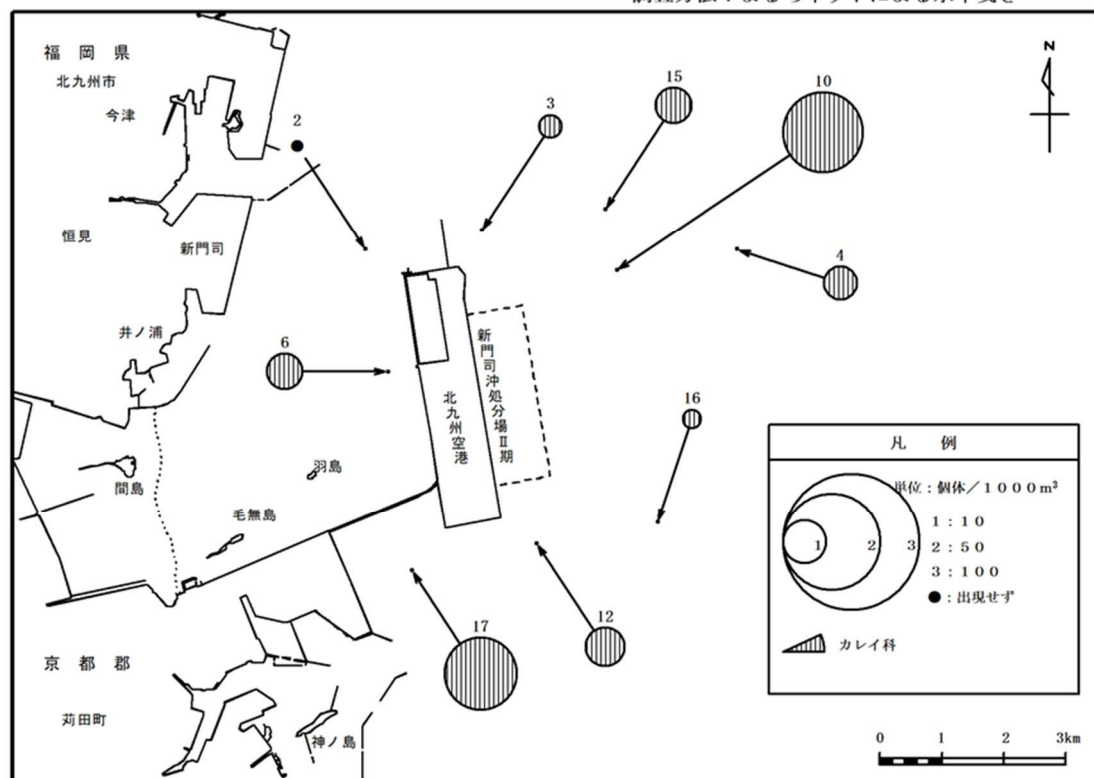
図 2. 2. 24(4) 魚卵の水平分布（令和 4 年度冬季）
