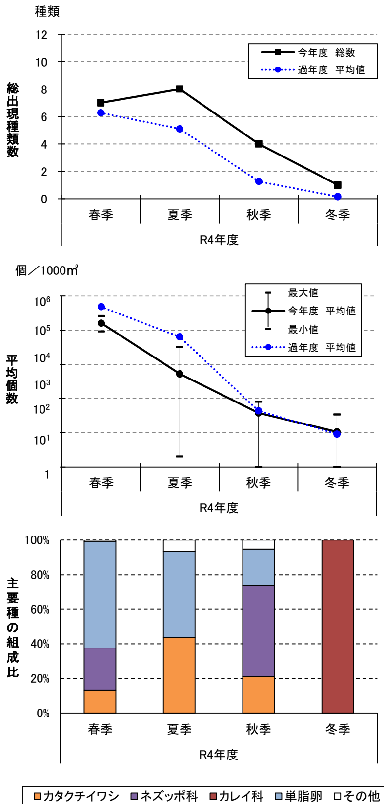
図 2.2.23 季節別出現状況図（魚卵）
