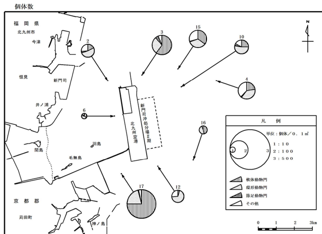
図 2.2.33 (4) 底生生物の水平分布（令和 4 年度冬季：種類数・個体数）
