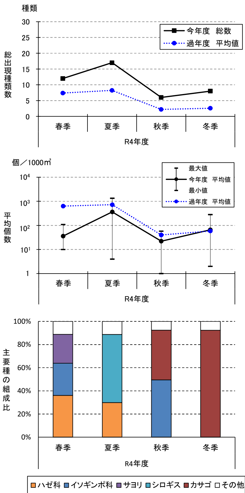
図 2.2.25 季節別出現状況図（稚仔魚）
