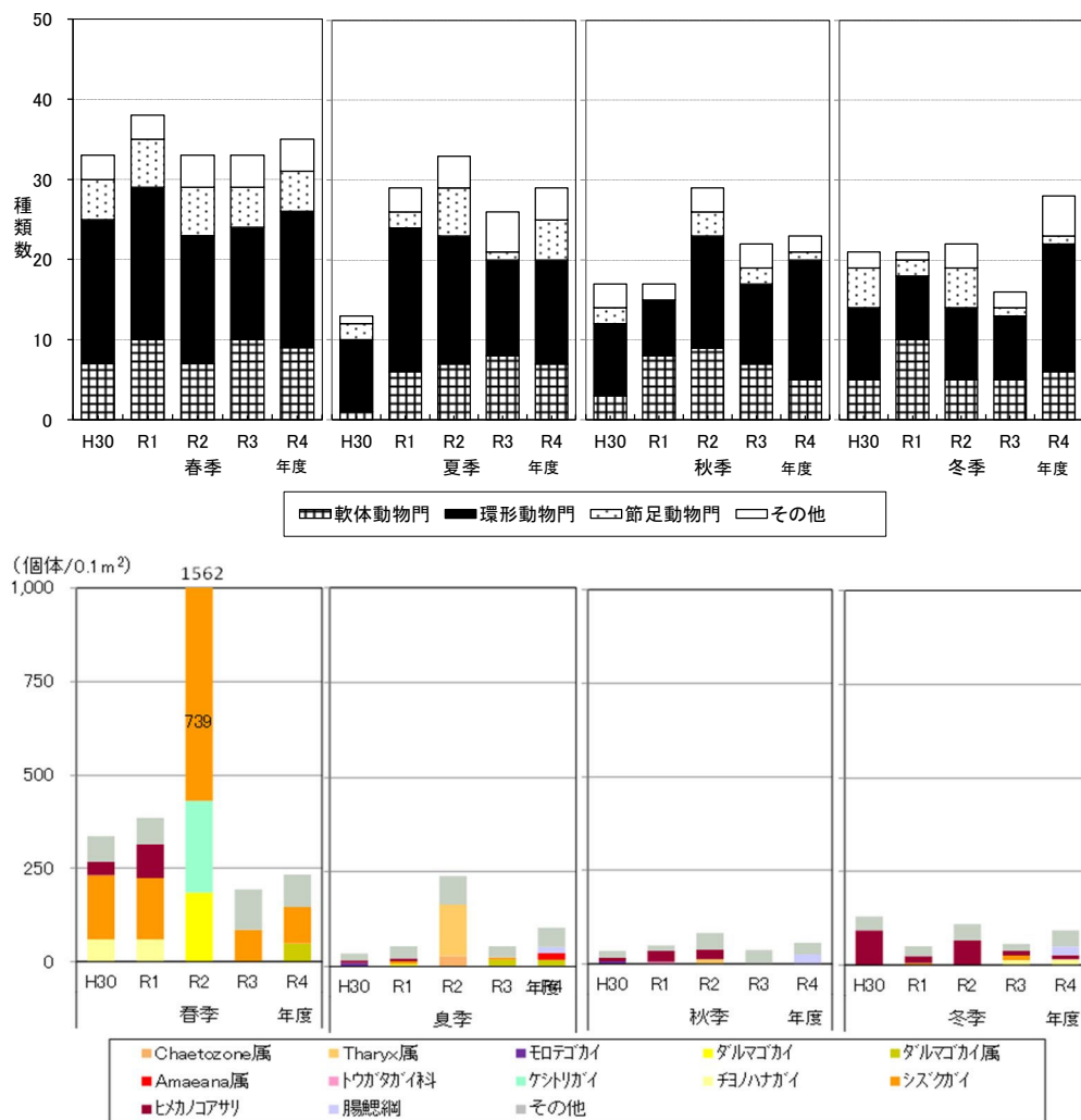
図 2.2.34(7) 底生生物の経年変化 (No. 15)
