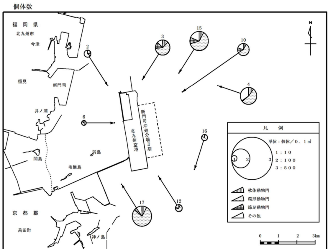
図 2.2.33 (2) 底生生物の水平分布（令和 4 年度夏季：種類数・個体数）
