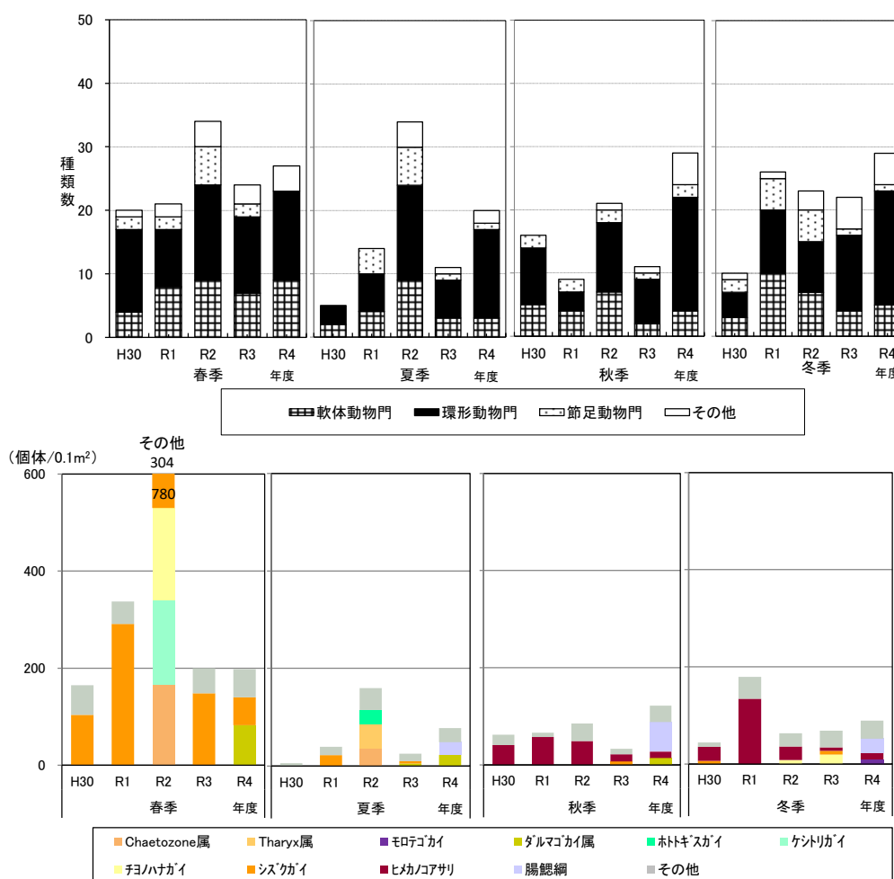
図 2.2.34(3) 底生生物の経年変化 (No. 4)
