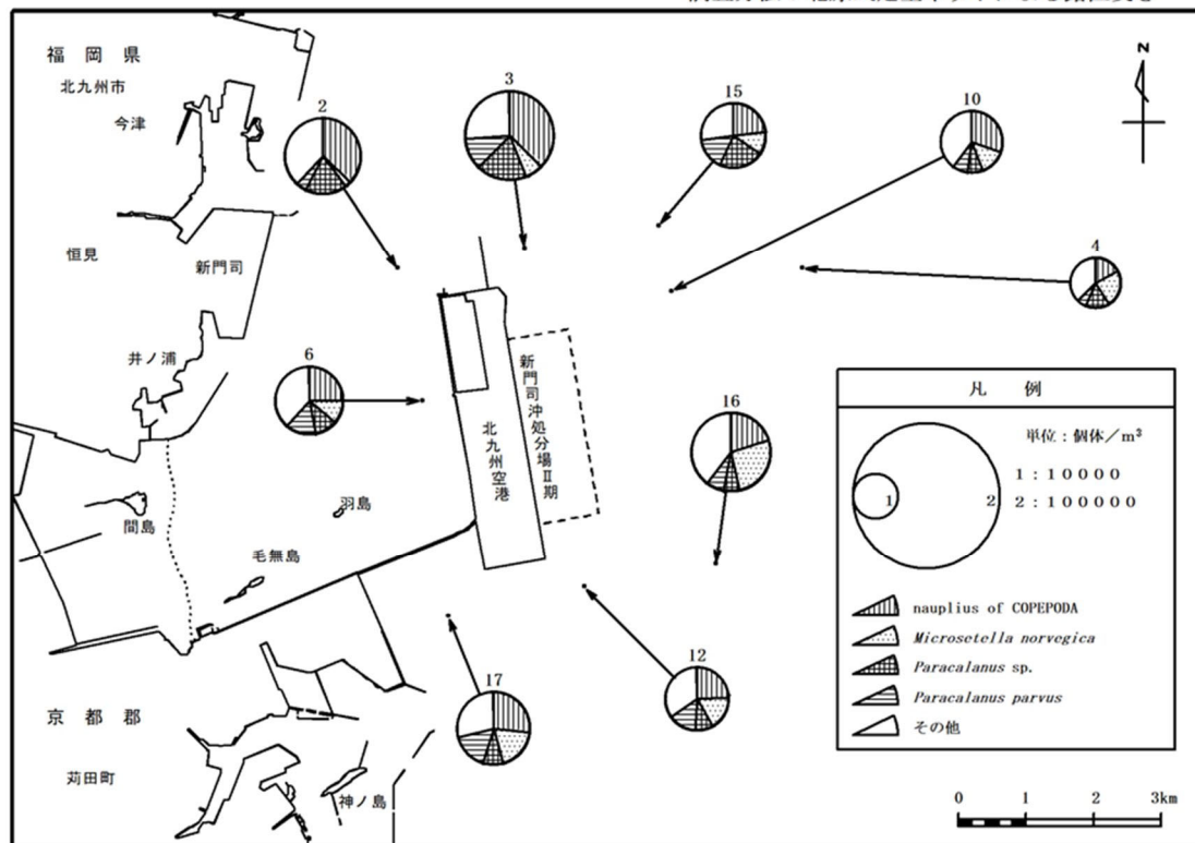
図 2.2.20(4) 動物プランクトンの水平分布（令和 4 年度冬季）
