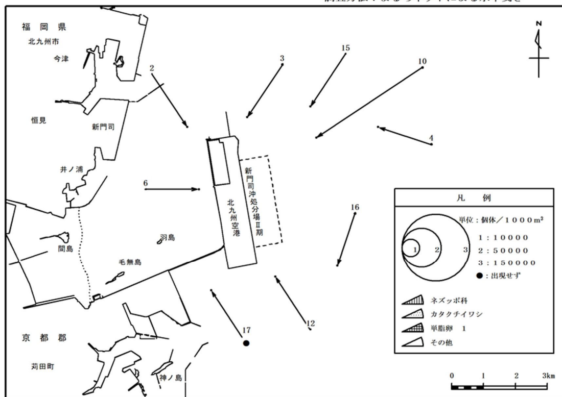
図 2. 2. 24(3) 魚卵の水平分布（令和 4 年度秋季）
