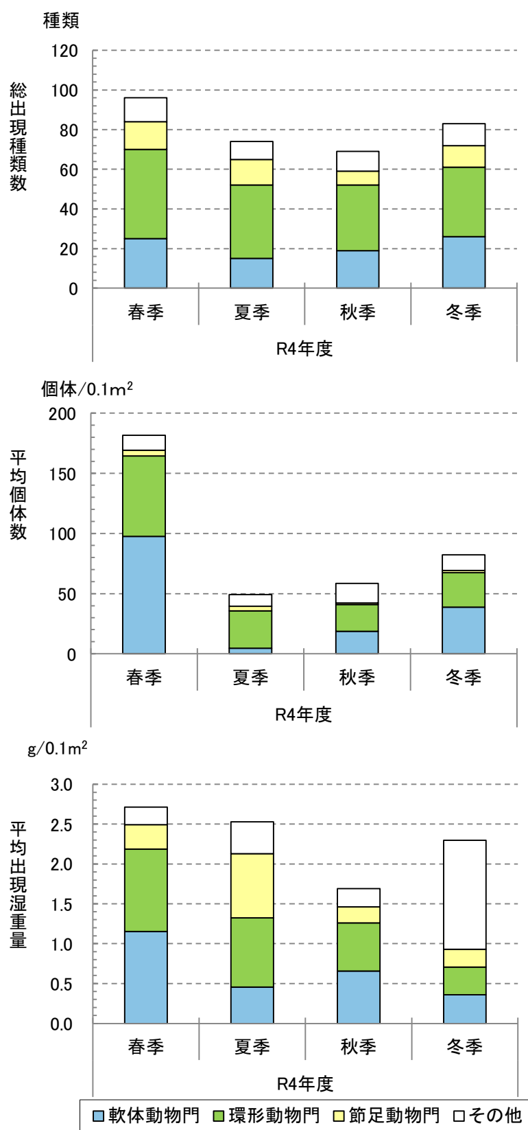
図 2.2.31 季節別出現状況図（底生生物）
