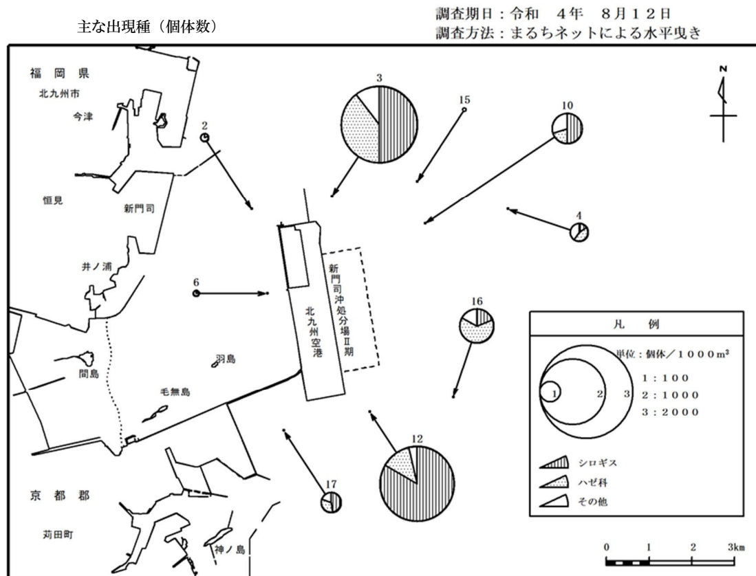
図 2.2.26(2) 稚仔魚の水平分布（令和 4 年度夏季）
