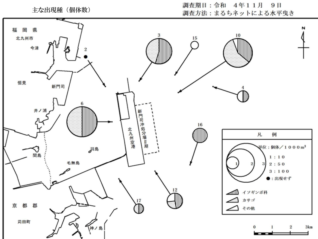
図 2.2.26(3) 稚仔魚の水平分布（令和 4 年度秋季）
