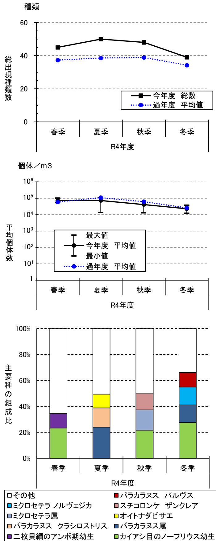
図 2.2.19 季節別出現状況図（動物プランクトン）
