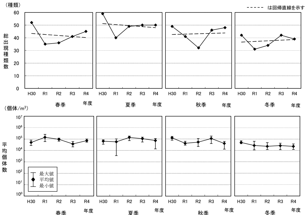
図 2.2.21 動物プランクトンの経年変化
