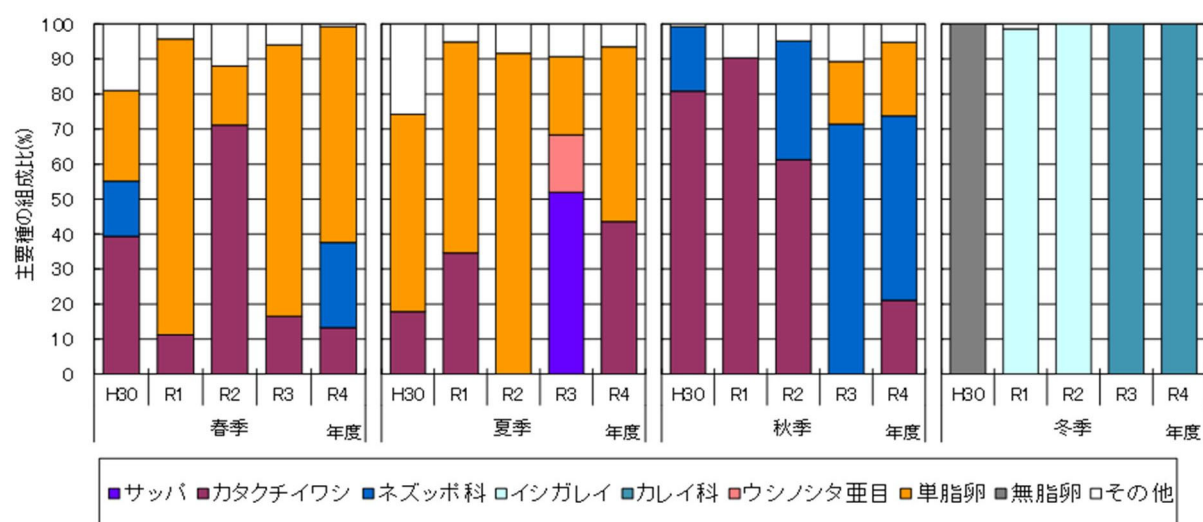
図 2.2.28 主な出現種の経年変化 (魚卵)
