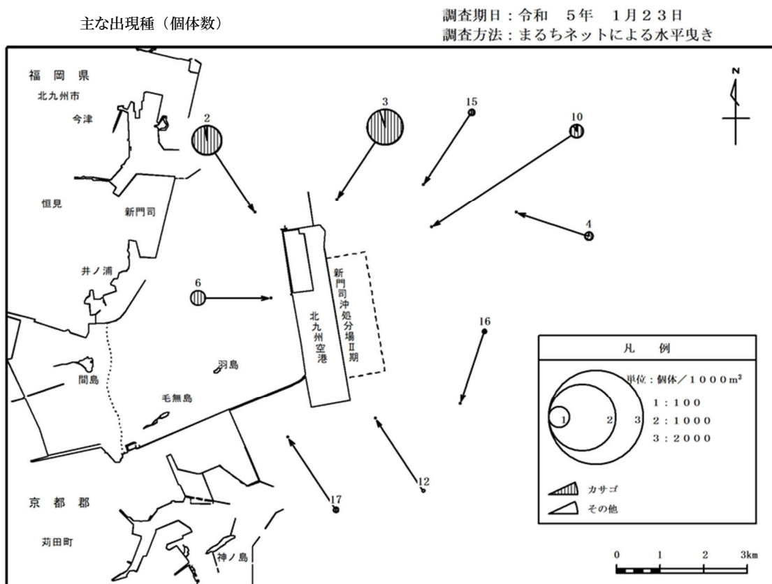
図 2.2.26(4) 稚仔魚の水平分布（令和 4 年度冬季）
