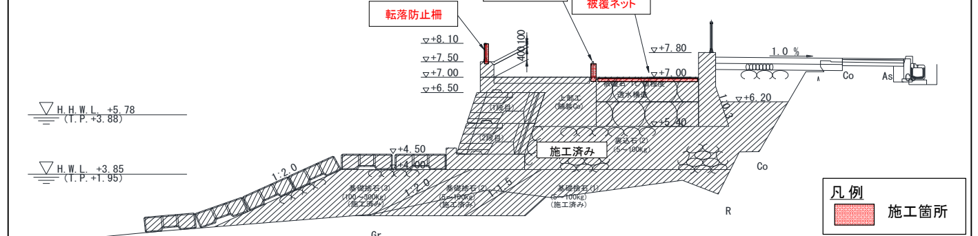
図-6 断面図(工事箇所③)
