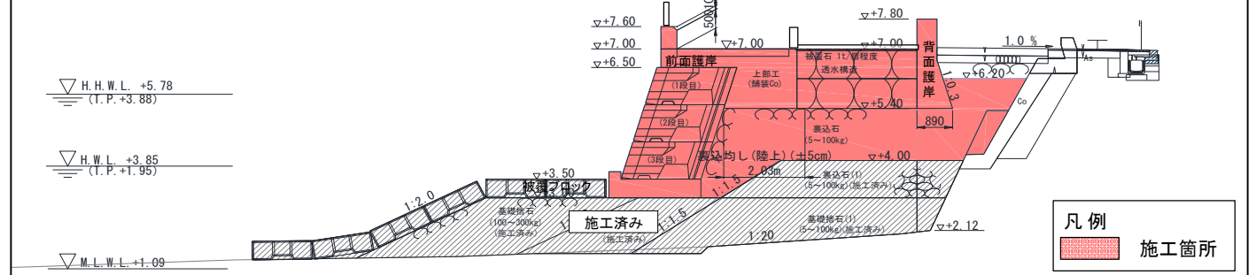
図-2 断面図(工事箇所①)
