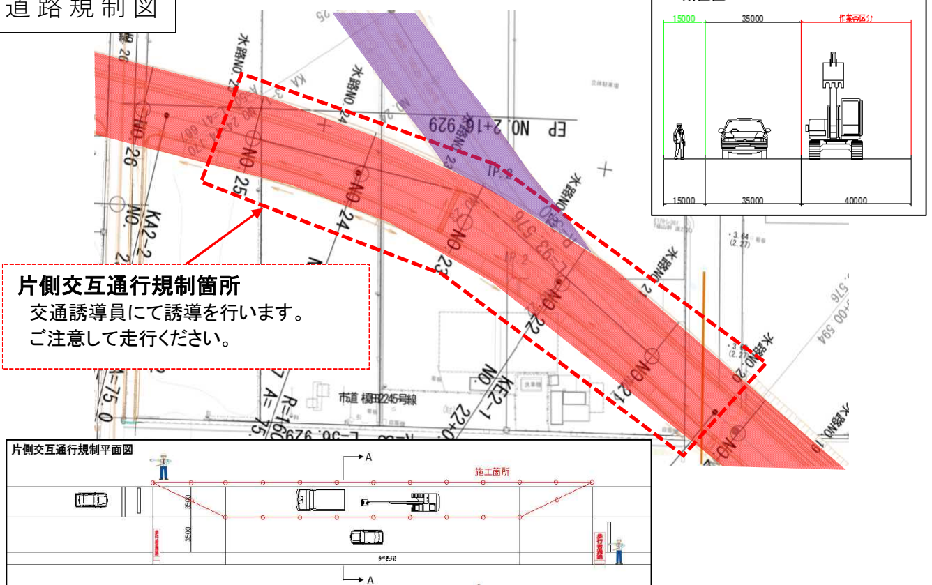
道路規制図
