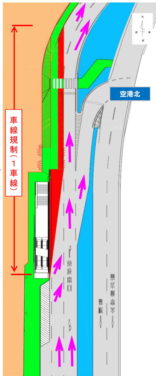
車線規制図
