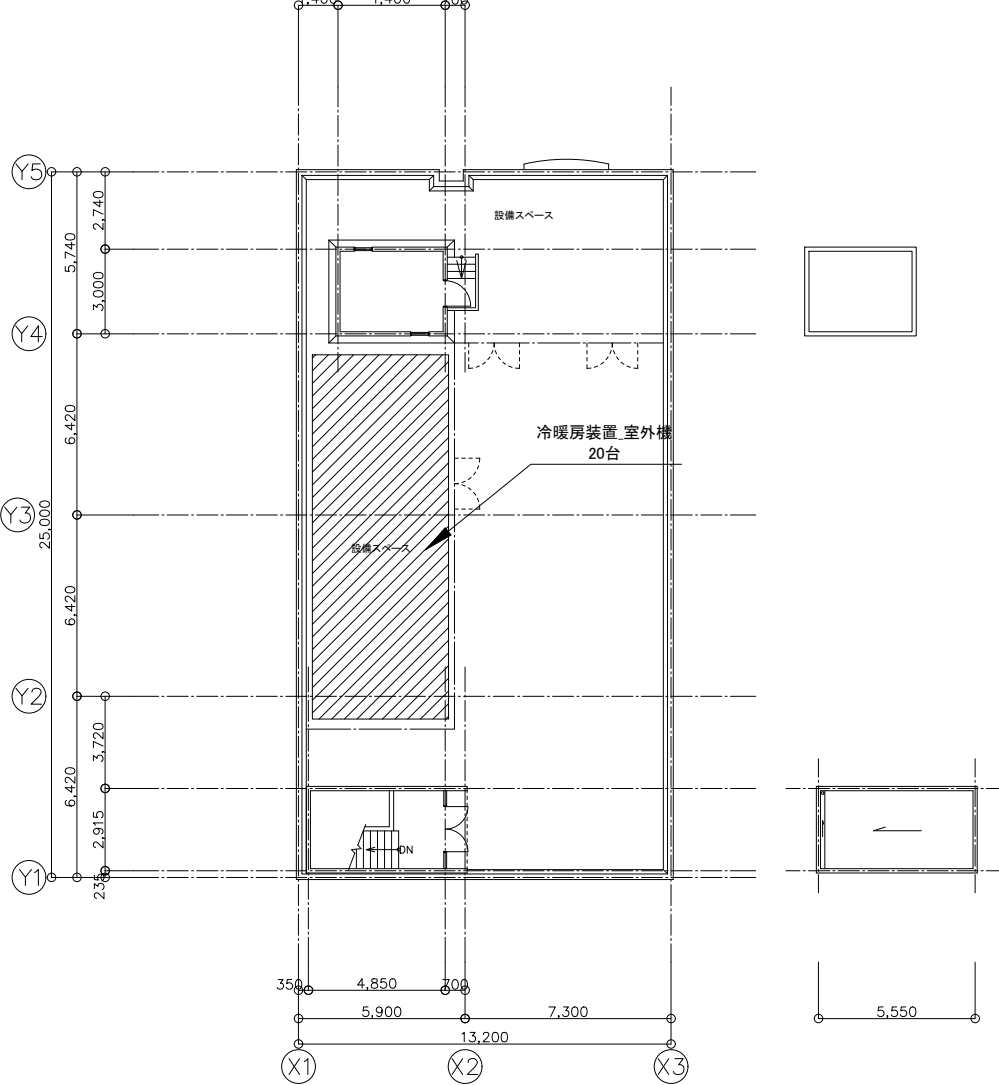
庁舎5階・塔屋階平面図
