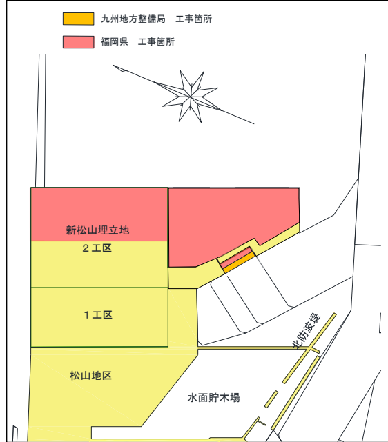
図-2 工事箇所及び作業区分
