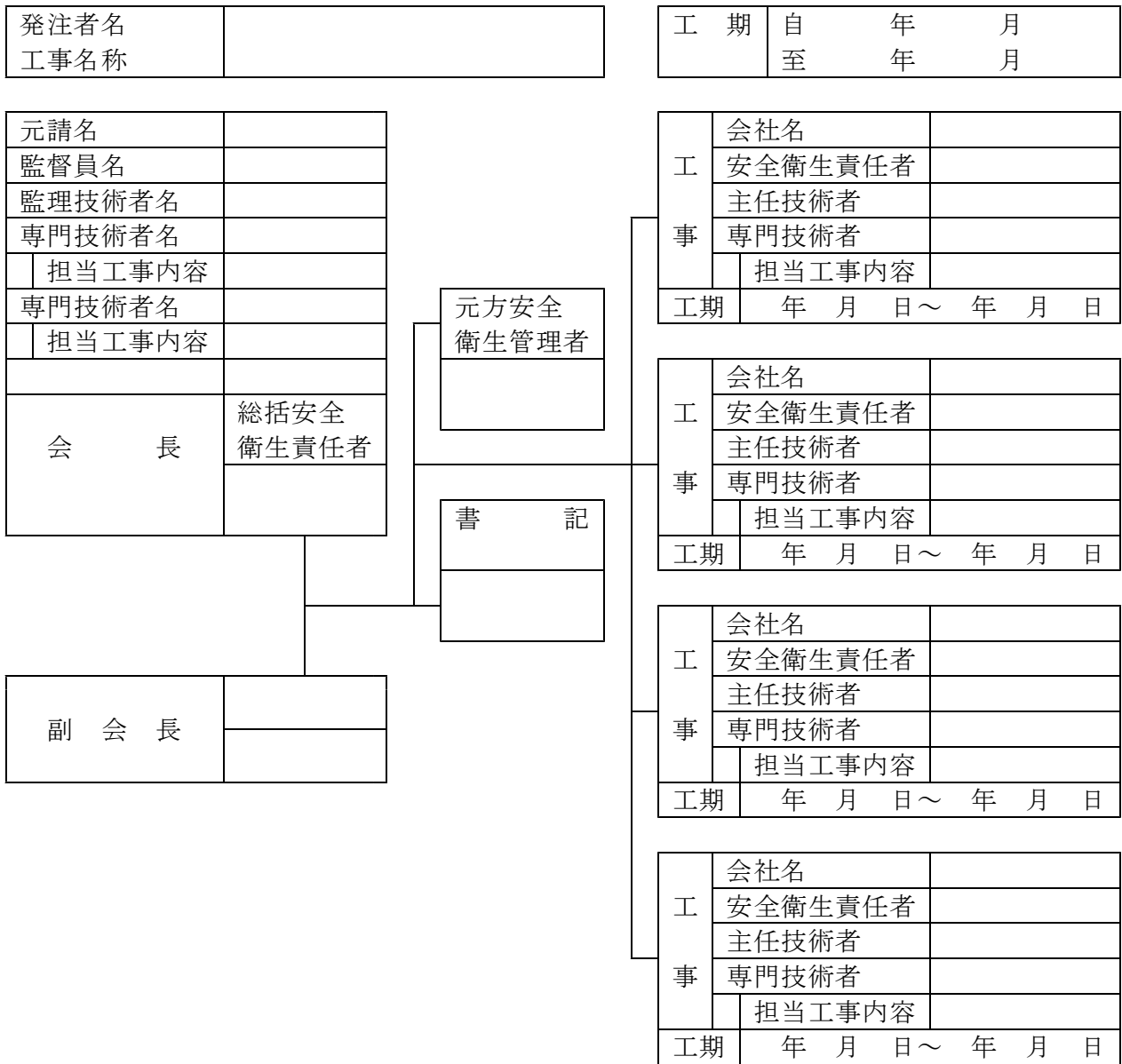
工事作業所災害防止協議会兼施工体系図
