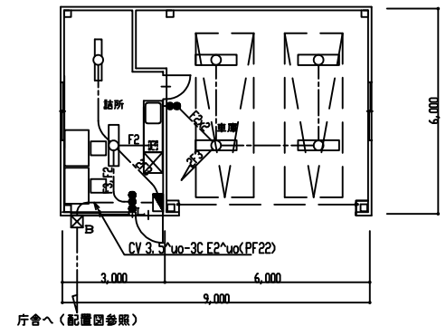
車庫平面図 1/100
