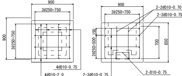
底板
