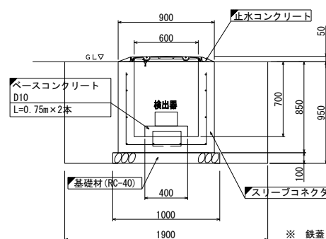
構造図 A3:1/50
