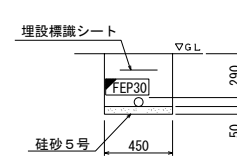
地中配管参考図
