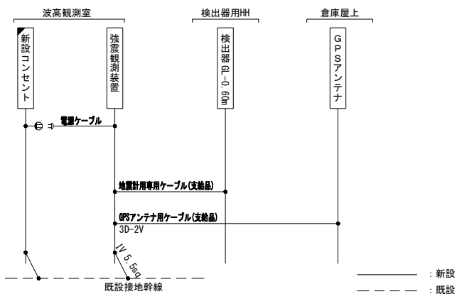
配線系統図
