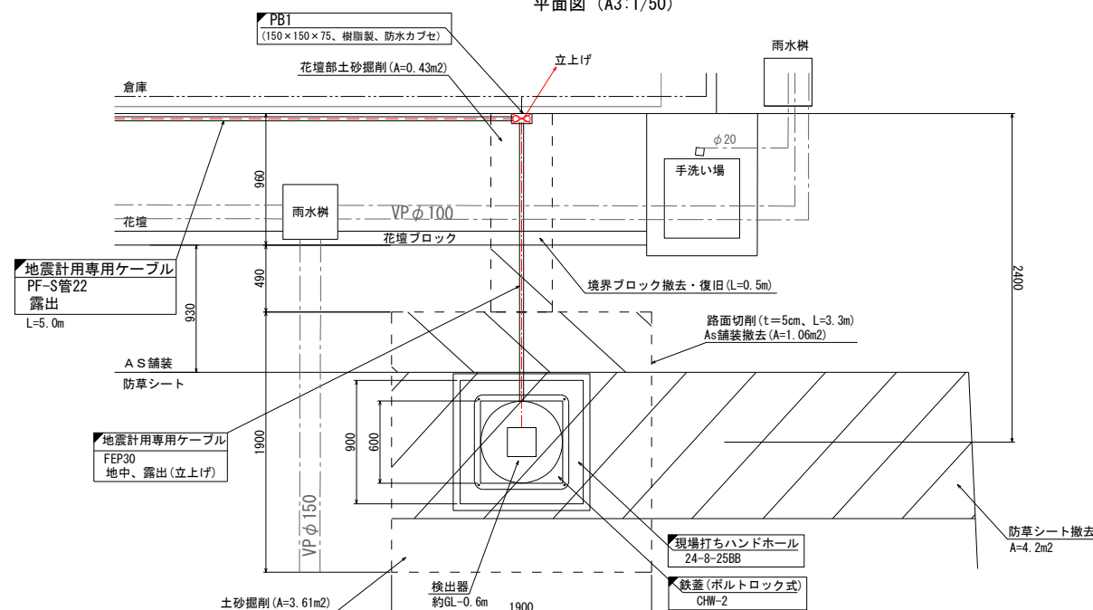
平面図 (A3:1/50)
