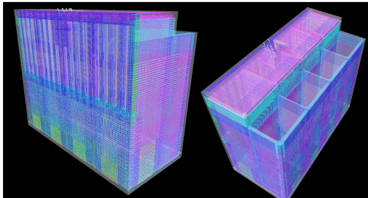
岸壁のケーソンのCIMモデル(構造物モデル)
