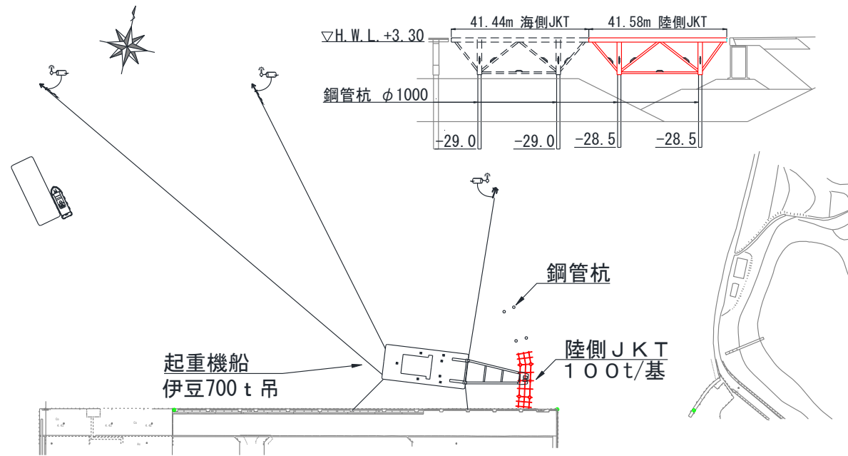
①ジャケット運搬作業
