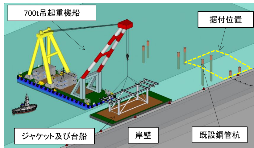
②据付準備作業
