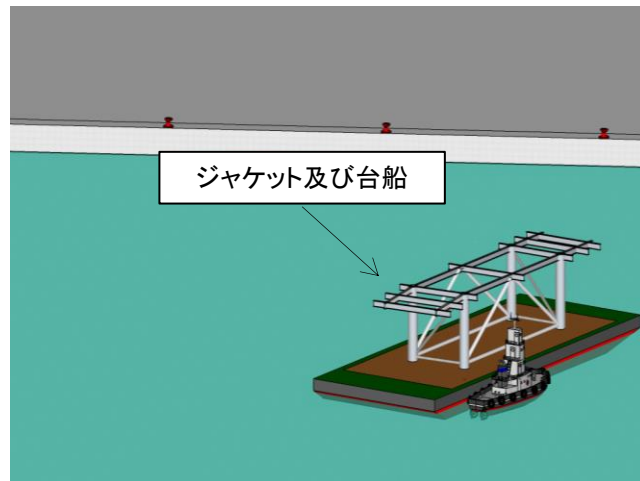
③据付作業
