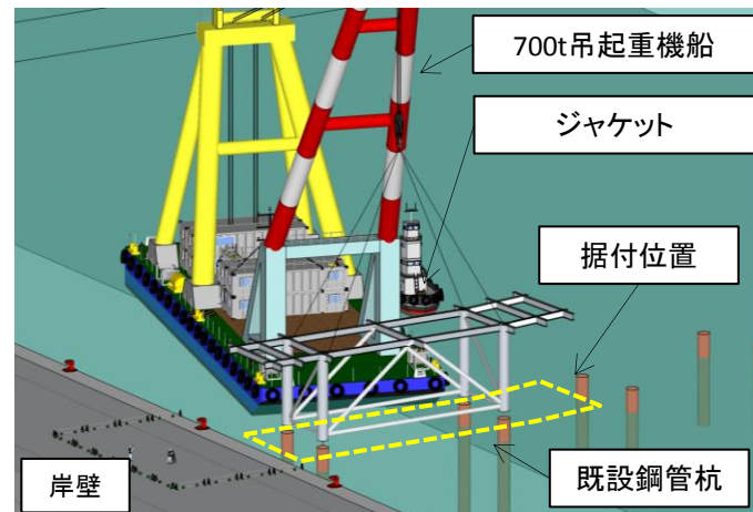
③据付作業
