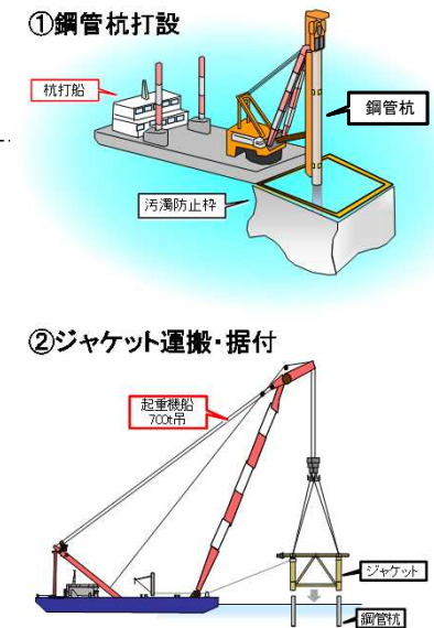
佐世保港(浦頭地区)国際クルーズ拠点整備事業 全体作業工程（現地作業）
