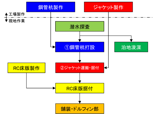
佐世保港(浦頭地区)国際クルーズ拠点整備事業 全体作業工程（現地作業）
