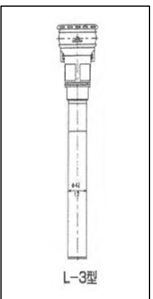
図-8 標識灯
