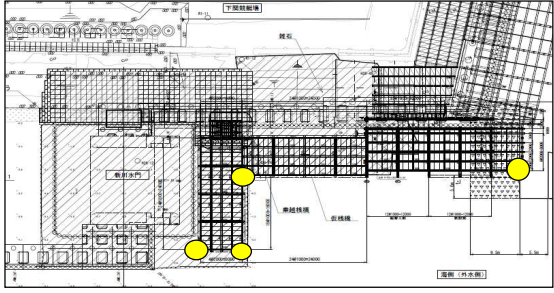
図-6 標識灯設置箇所(新川水門)
