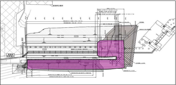
図-2 平面図(宮崎水門)
