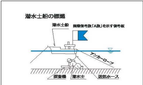
図-6 潜水探査概念図
