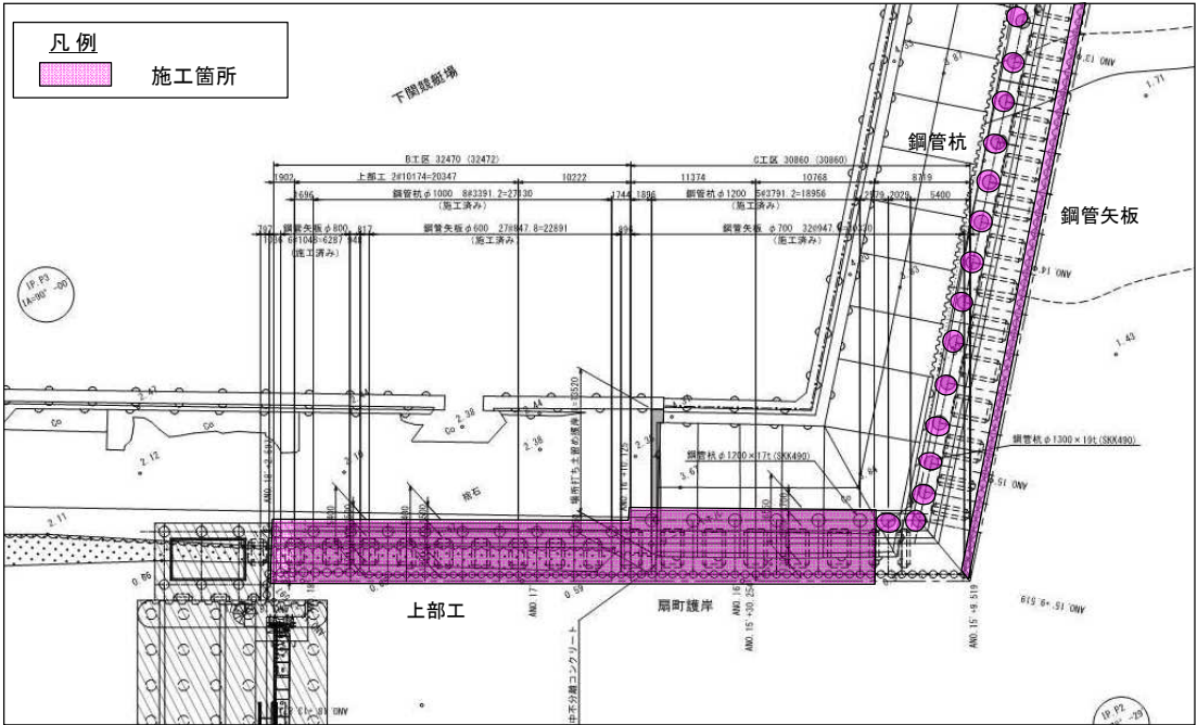
図-2 平面図(新川水門)
