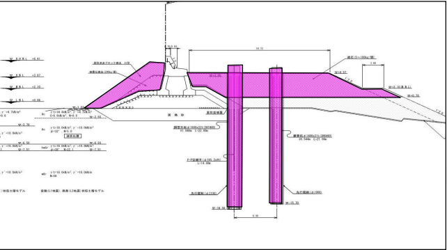
図-3 断面図(宮崎水門)
