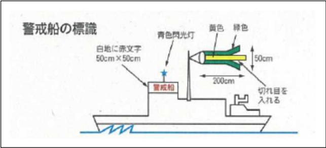
図-3 警戒船
