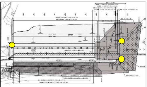
図-7 標識灯設置箇所(宮崎水門)
