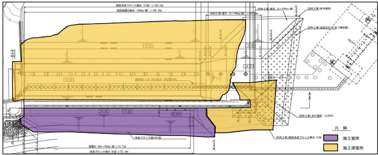
図-2 平面図(宮崎水門)
