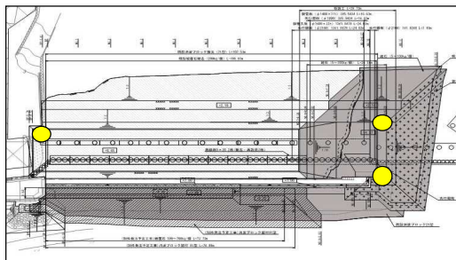
図-7 標識灯設置箇所(宮崎水門)
