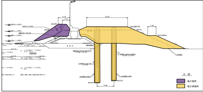
図-3 断面図(宮崎水門)
