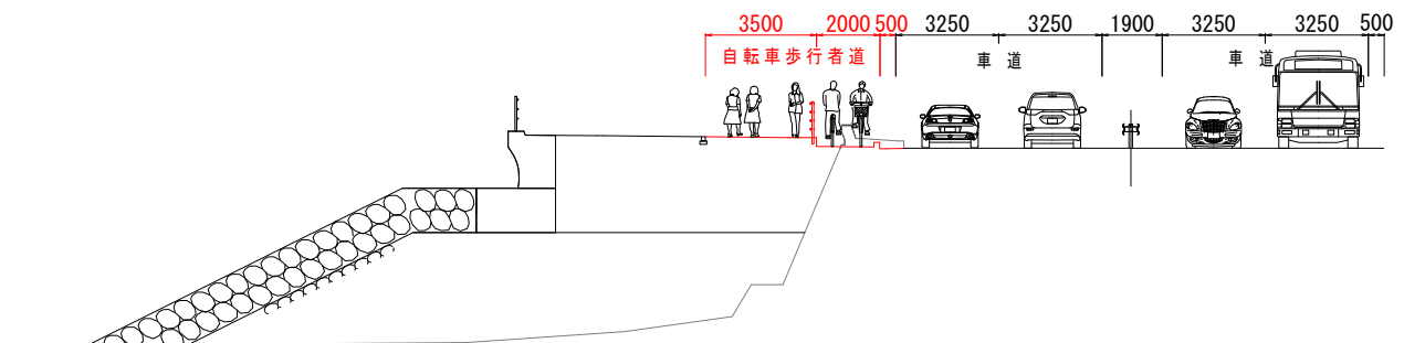
計画断面図
