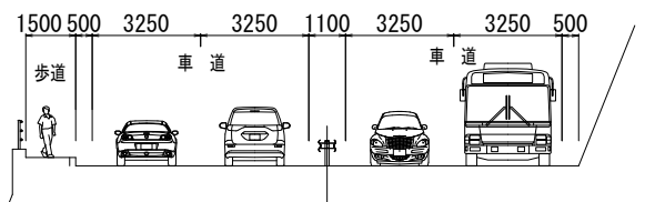
現況断面図
